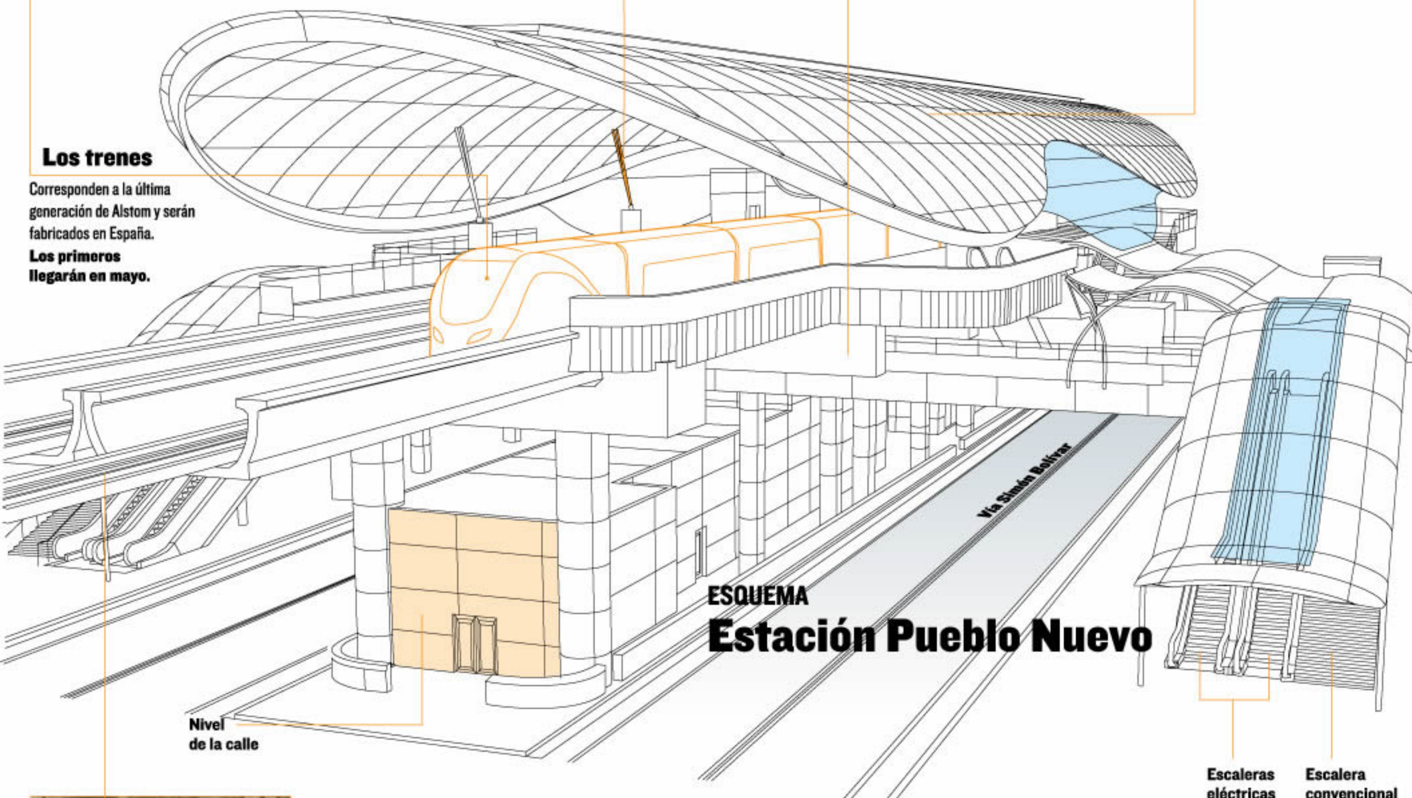
3 Armazón del techo
